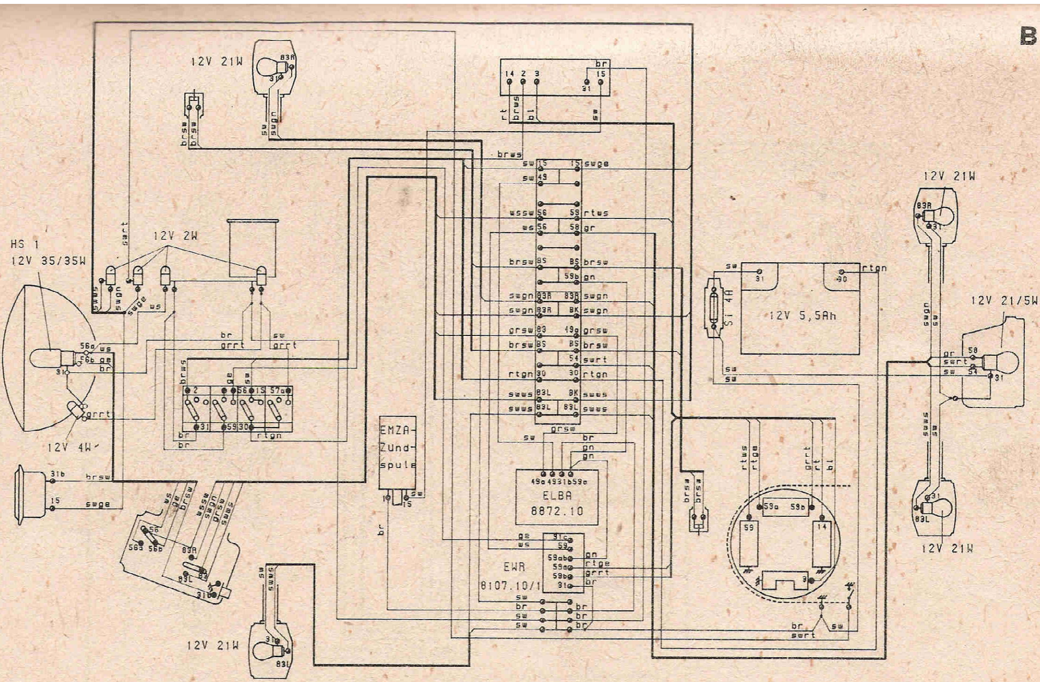
Bild 215. Schaltplan für SR 50/1 C
